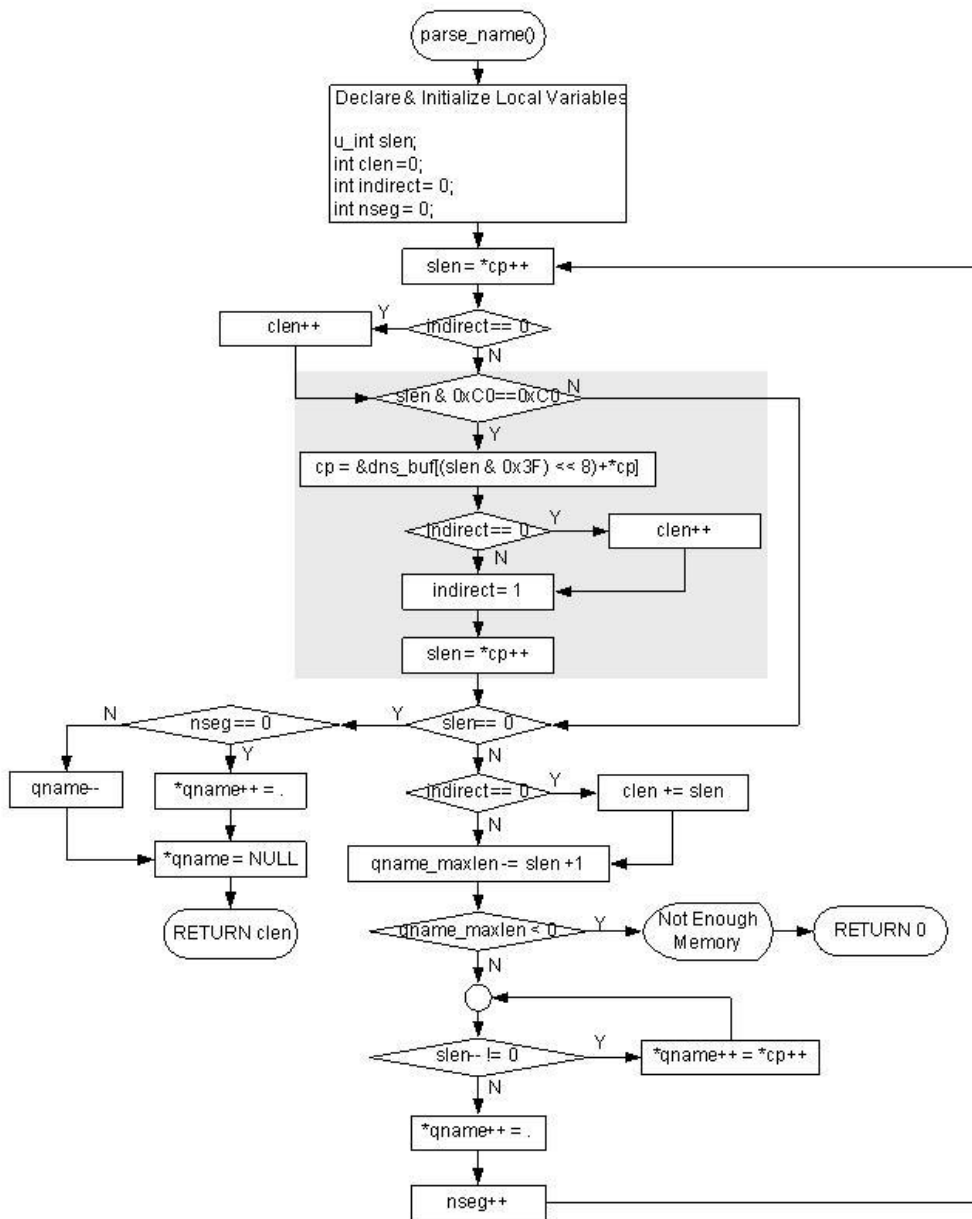
<Fig 3.44: parse_name()>
